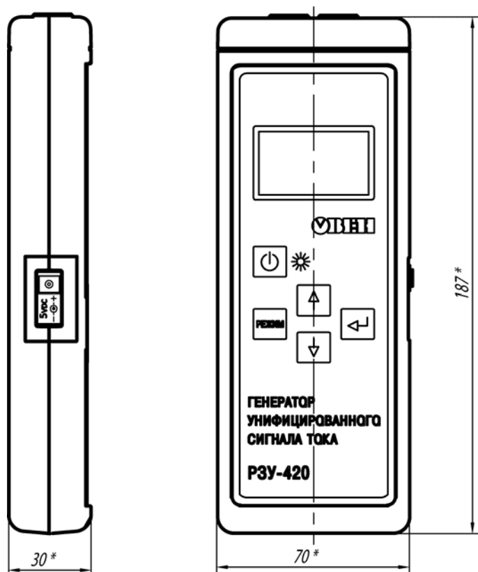
Рисунок А.1 – Габаритный чертеж прибора
