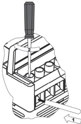
Рисунок 6.1 – Подключение провода к клемме
